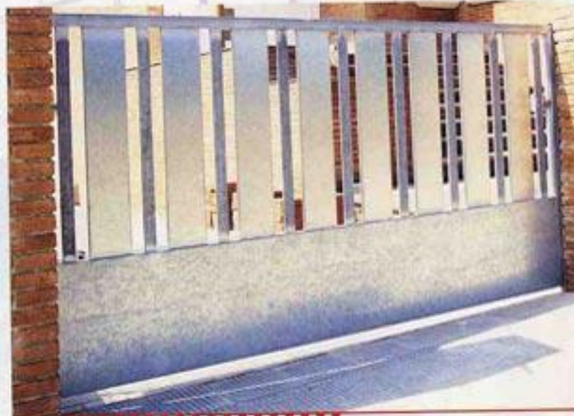
Porta practicable automàtica d'una sola fulla, folrada amb xapa galvanitzada doblada. L'acabat és amb barrots verticals i sòcol cec.
